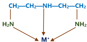
Diethylenetriamine(dien) Tridentate
